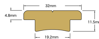
32 mm T トラック原寸図
