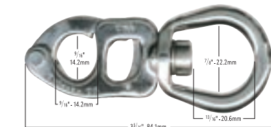
ラージペイル
