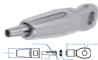
1×19 ワイヤー用アイターミナル
