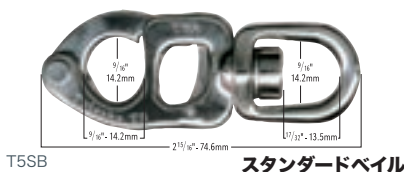
スタンダードペイル
