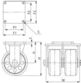
EUYW 重量型 固定キャスター
