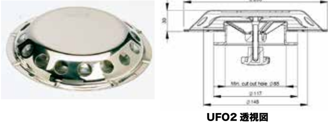
UFO2 透視図
