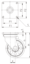
EUYO 重量型 自在キャスター
