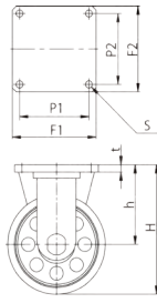
EUYW 重量型 固定キャスター
